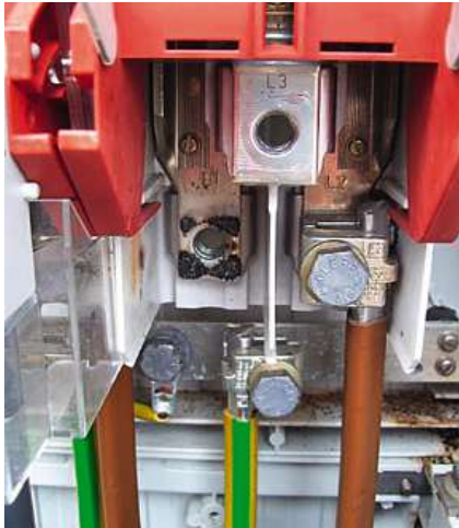
Bild 6 Mangelhafte Verschraubung.
