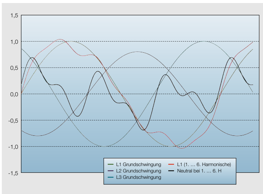
Bild 1 Neutralleiterspannung (schwarz) bei überschwingungsbehaftetem 3-Phasensystem mit Schiefelast.
