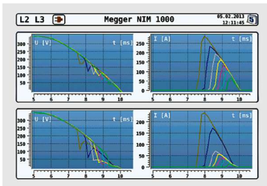
Bild 5 Fehlerfreie Verbindung (oben) und fehlerbehaftete Phase (unten).
