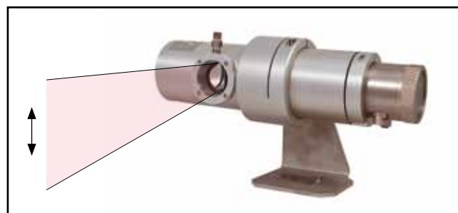
Capteur Endurance installé dans un SpotScan équipé d'une purge à air (en option)
